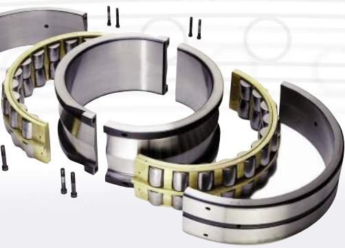
Roulement à rotule sur deux rangées de rouleaux en deux parties
