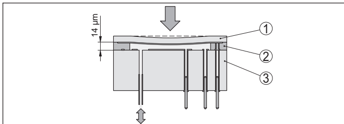
Fig. 1: Structure de la cellule de mesure Mini-CERTEC®
