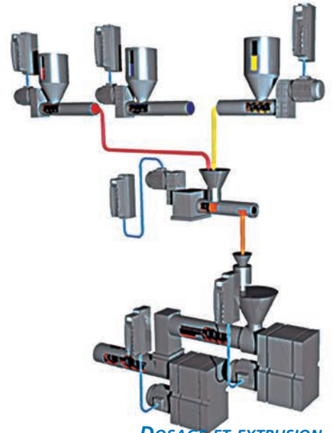
DOSAGE ET EXTRUSION
