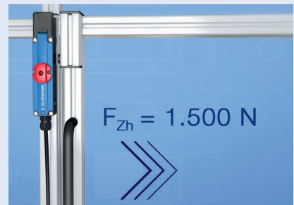
Force de verrouillage élevée Conception mince et force de verrouillage élevée F_{Zh} = 1.500 \text{ N}
