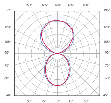
PHOToméTRIE MODULE ÉCLAIRAGE DIRECT/INDIRECT
