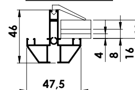
Profil de parois et de toit
