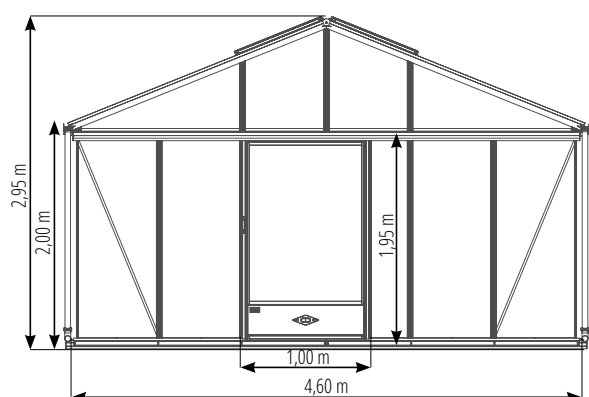
Structure avec profils renforcés et entrants pour les longueurs 6,78 m, 7,53 m et 8,30 m
