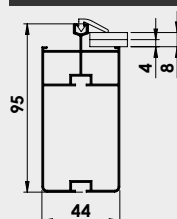
Profil de toit pour profondeurs 2,32 m et 3,06 m
