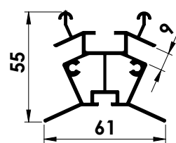
Profil de parois et de toit
