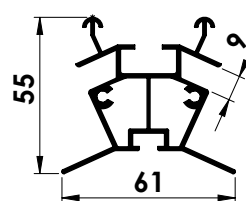
Profil de faîtage
