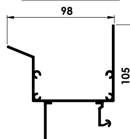
Profil de gouttière
