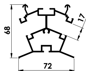
Profil de gouttière
