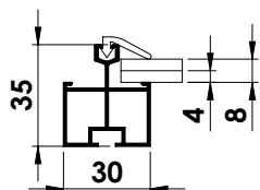
Profil de parois et de toit
