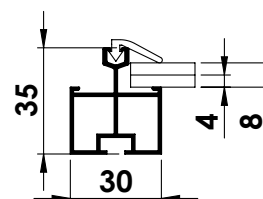
Profil de parois et de toit
