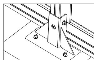
Sabot de renfort
