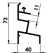
Profil de gouttière
