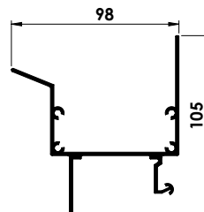
Profil de gouttière
