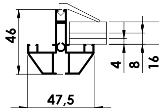
Profil de parois et de toit
