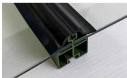
Équipement standard : joint EPDM
