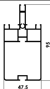
Profil renforcé de parois et de toit
