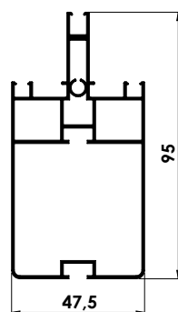
Profil renforcé de parois et de toit
