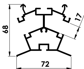
Profil de faîtage
