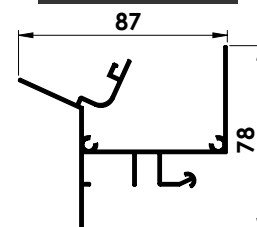
Profil de parois et de toit
