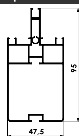
Profil renforcé de parois et de toit
