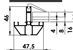
Profil de parois et de toit
