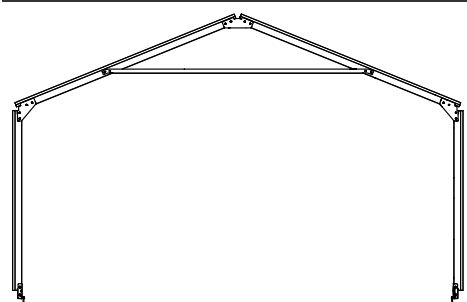
Structure avec profils renforcés et entrants pour les longueurs 6,78 m, 7,53 m et 8,30 m
