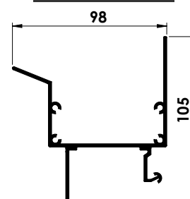
Profil de gouttière
