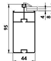
Profil de toit pour profondeurs 2,32 m et 3,06 m
