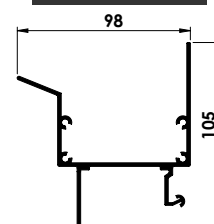
Profil de gouttière
