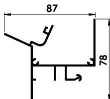
Profil de gouttière
