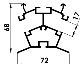
Profil de faîtage
