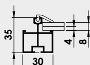
Profil de parois pour les 3 profondeurs & profil de toit pour la profondeur 1,58 m
