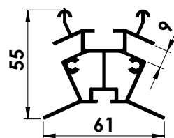
Profil de faîtage
