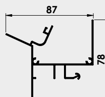
Profil de gouttière
