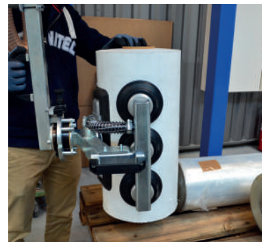
Manipulation de bobines par ventouses
