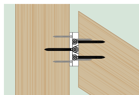
Assemblage oblique (vue de dessus)
