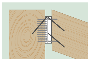
Assemblage incliné (vue de côté)
