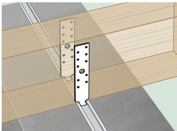
Exemple d'application SXPA dans rail Halfen
