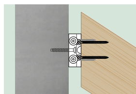
Assemblage oblique (vue de dessus)
