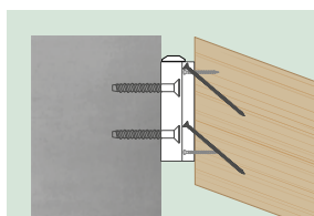
Assemblage incliné (vue de côté)
