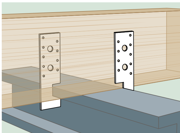
Exemple d'application SXHE sur poutre en acier
