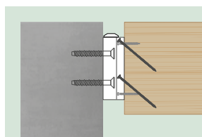
Assemblage 90° (vue de côté)
