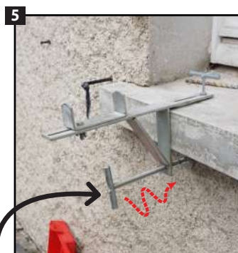
Serrer la pièce contre le crépi pour faire contrepois.
