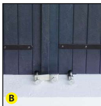
Déport du volet à l'aide de blocs polystyrène (voir photo n° 7).
