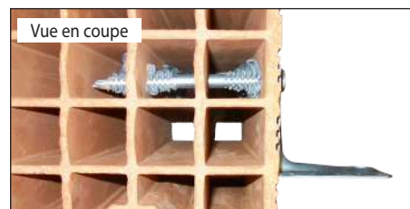
Lisse de bardage
