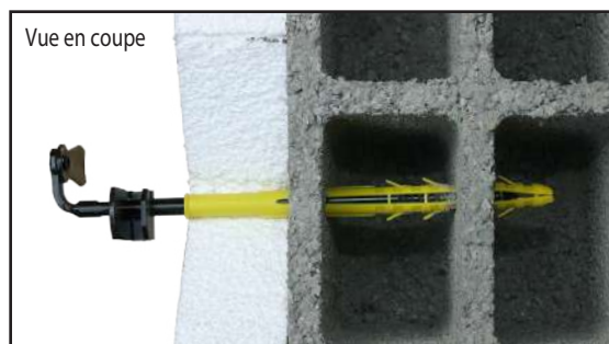
Dans le parpaing, expansion sur les deux alvéoles.
