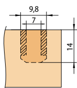
Profondeur de fraisage FIYU® FAST 14
