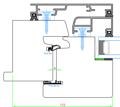
JEU DE 4MM - JOINTS SUR DORMANT
