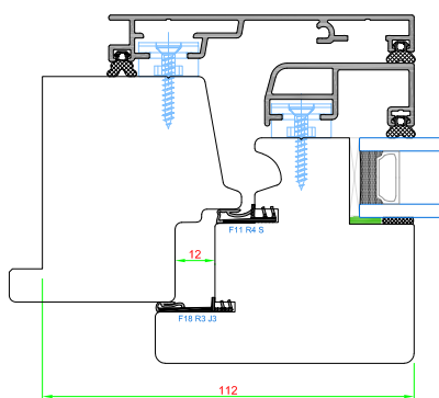
JEU DE 12MM - JOINTS SUR OUVRANT
