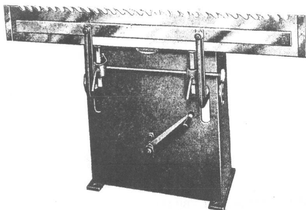
58-G Etau à écraser pour lames de châssis.
