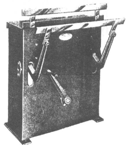
58-B-32 Etau à écraser pour lames à ruban mâchoires de 800 mm.
