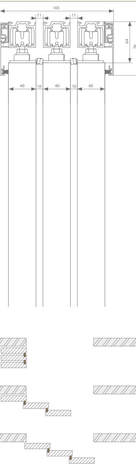
Parallel fixation au plafond 2
