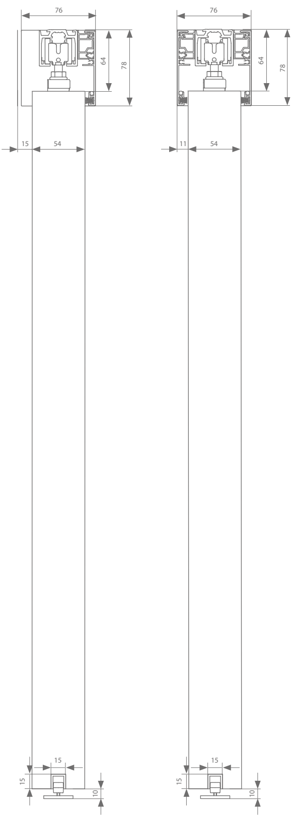
fixation au plafond 54 mm
