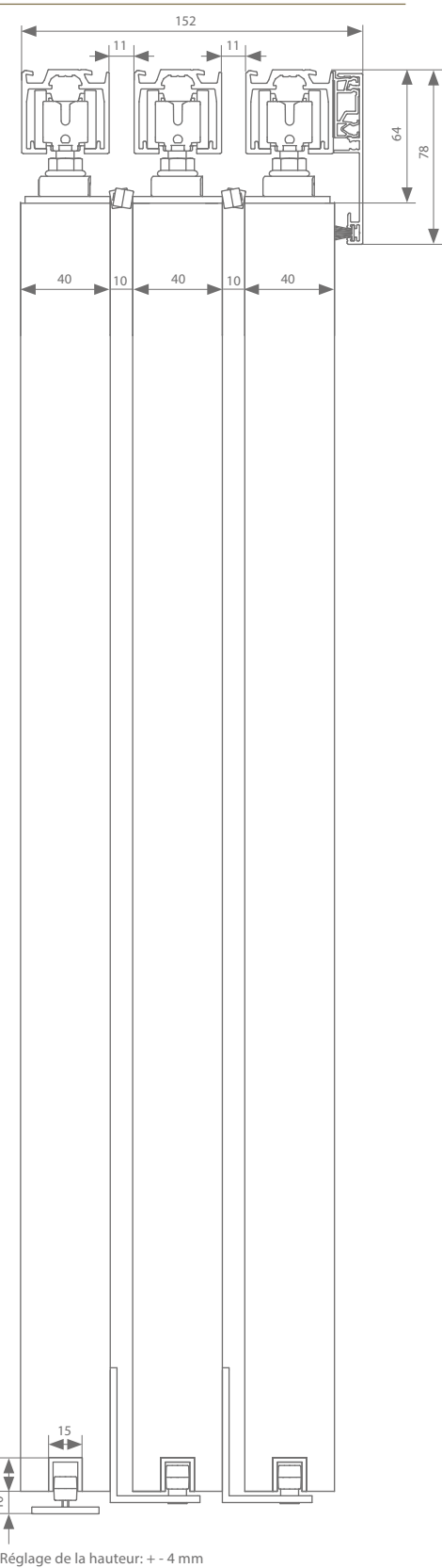
Parallel fixation au plafond 1
