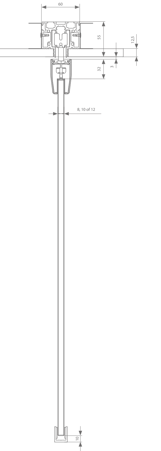
Réglage de la hauteur: +0 / - 5 mm
