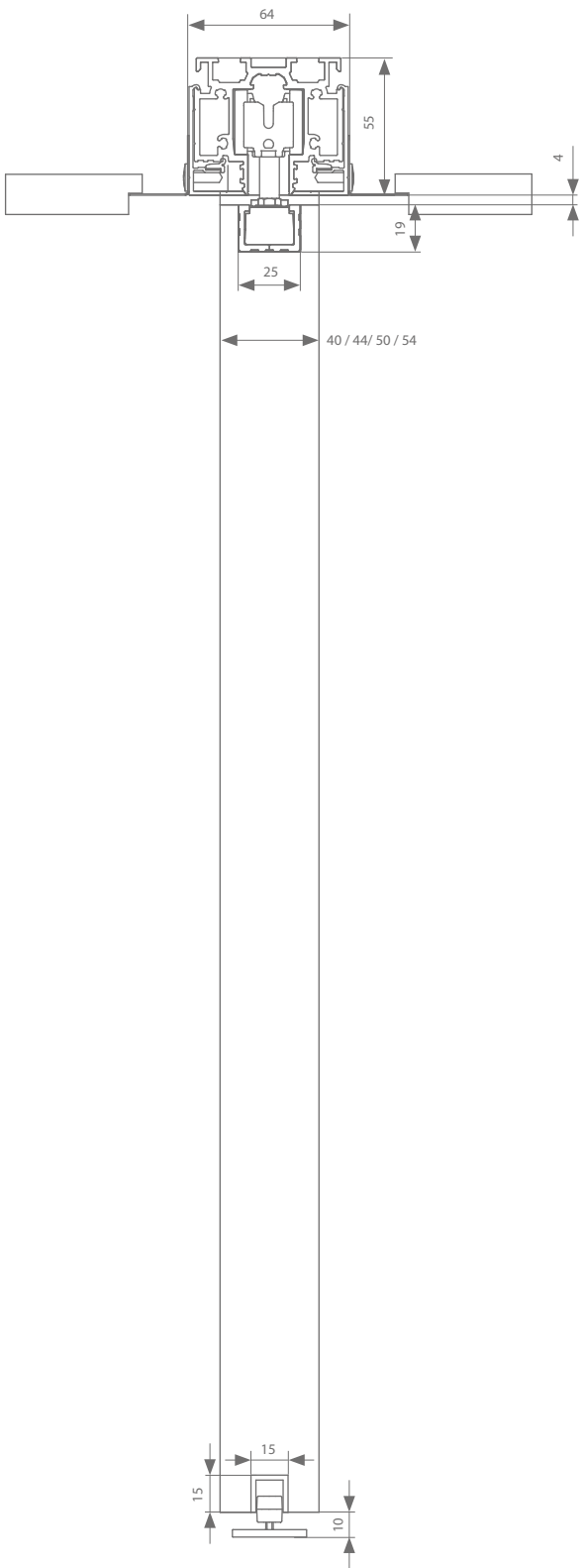
Pour plafond technique
