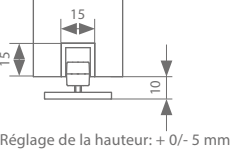
Réglage de la hauteur: + 0/- 5 mm
