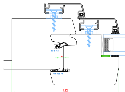
JEU DE 4MM - JOINTS SUR DORMANT
