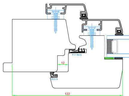
JEU DE 12MM - JOINTS SUR OUVRANT
