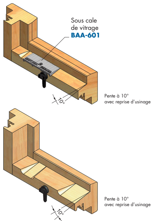
FEUILLURE À VERRE EXTENSIBLE
