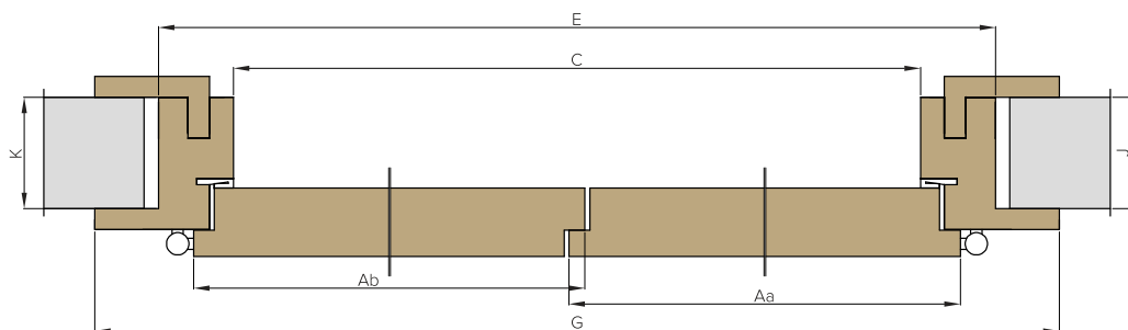
Double vantail avec feuillure avec huisserie réglable
