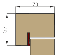
coupe 57 x 70 mm
