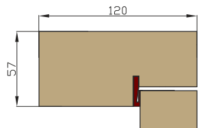
coupe 57 x 120 mm
