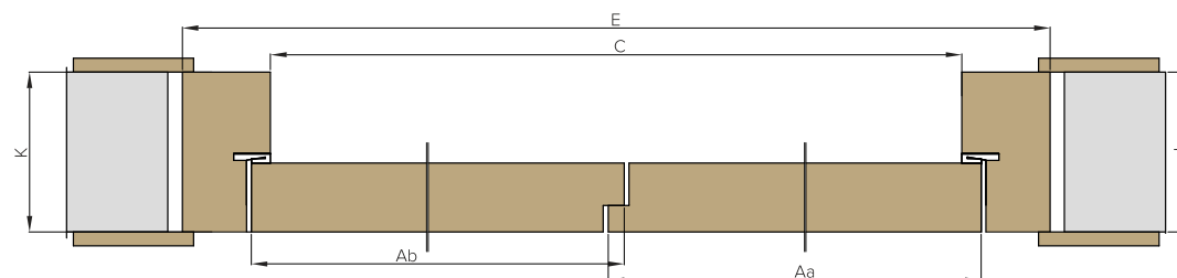
Double vantail sans feuillure avec huisserie fixe
