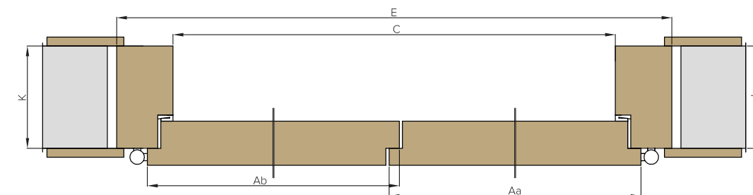
Double vantail avec feuillure avec huisserie fixe
