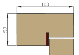
coupe 57 x 100 mm
