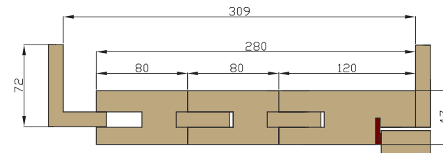
Plage de réglage "J" : 280 mm -309 mm
