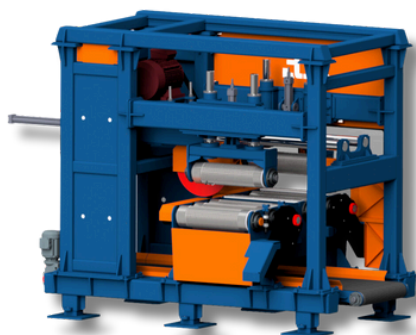
TRONÇONNEUSE À NOYAUX
