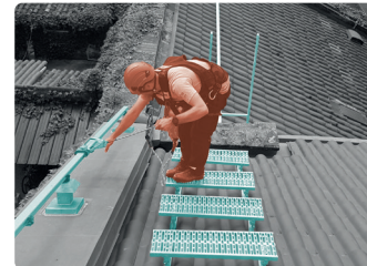
Mise en service d'une sécurisation complète, sur les toitures d'une MAIRIE .
