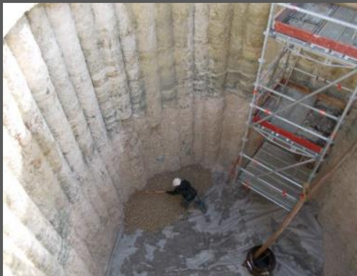
PIEUX SECANTS
