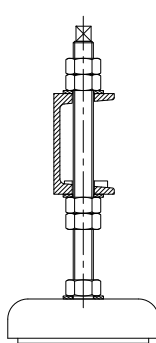
Pieds réglables sous la plaque de base
