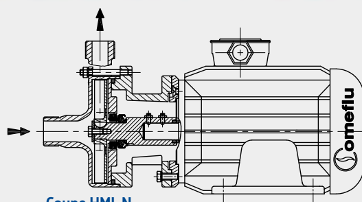
Coupe HMI-N avec garniture mécanique
