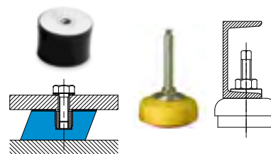
Isolateur de vibrations de la plaque de base et coussinets anti-vibrations
