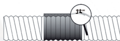
SCHEMA DE RACCORDEMENT DE 2 TUBAO® À L'AIDE D'UN COLLIER
