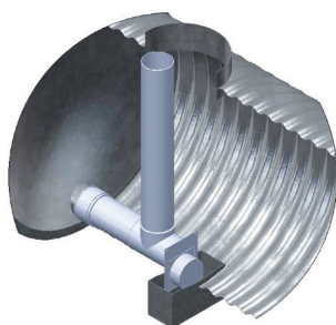
Trop plein intégré Version avec régulateur de débit extractible et marnage
