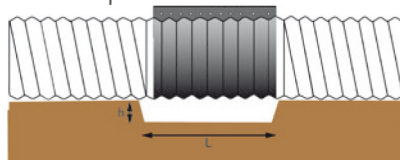
SCHEMA D'UN DÉCAISSEMENT SOUS COLLIER
