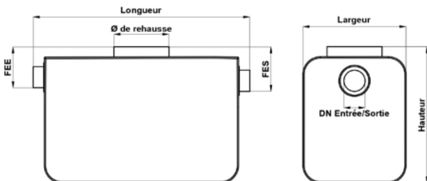
Schéma d'un séparateur hydraulique
