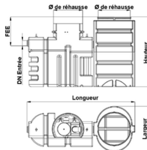
Schéma d'un OleocidoLift
