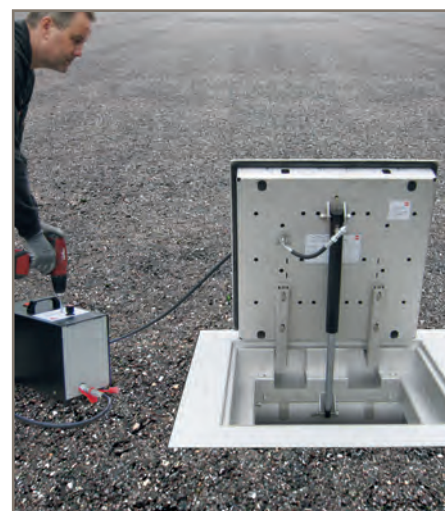
Capots à ouverture hydraulique
