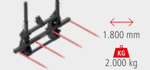
GRIFFE À BALLES BGZ
