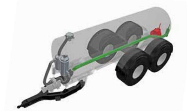
Tracé de conduite, vidange en descente de la tonne à lisier sous vide
