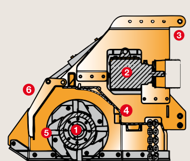
Marteaux fixes BPN
