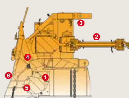
Marteaux mobiles BP - BPR
