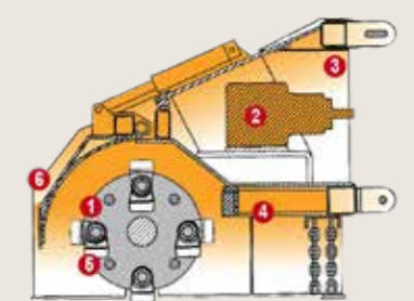
Marteaux mobiles BP - BPR
