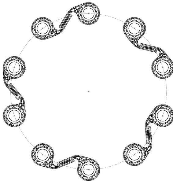
Exemple sur entreaxe 335mm, 10 écrous
