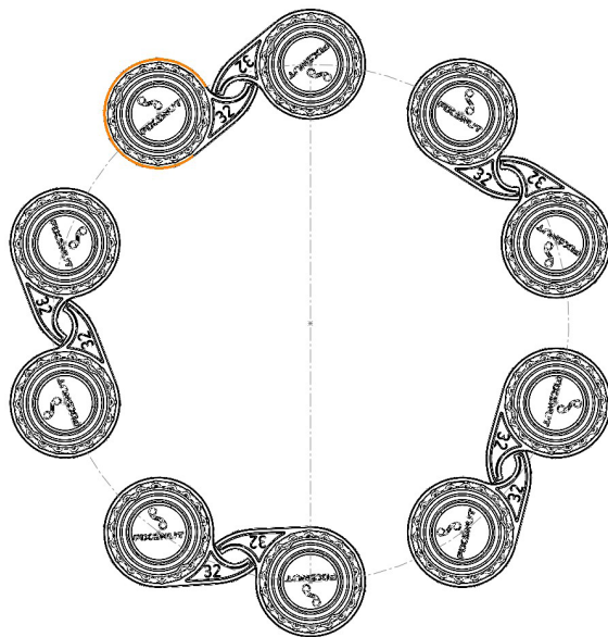
Exemple sur entraxe 225mm, 10 écrous
