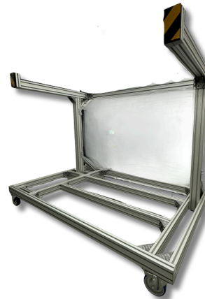
Chariot spécial en profilés aluminium pour transport de racks
