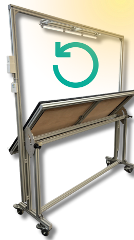
Plan de travail avec option inclinaison et éclairage sur batterie
