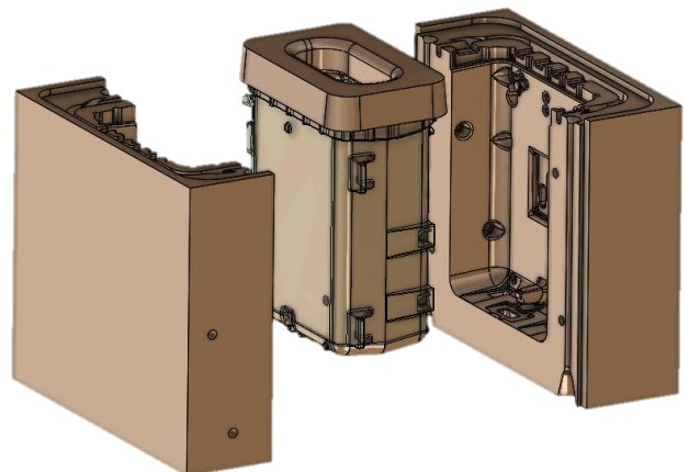
Etude fonderie
