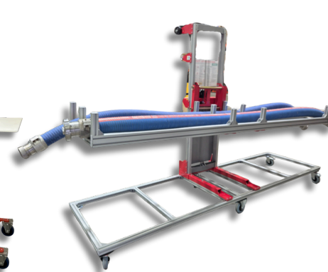
Gerbeur sur mesure pour manipulation de flexibles
