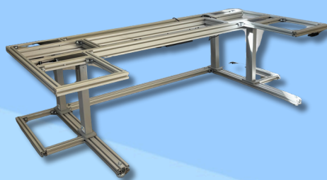
Plan de travail réglable électriquement en hauteur, conçu en profils aluminium
