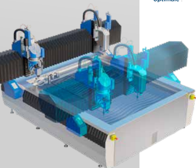
- Configuration Double Pont, modèle WJA II 30.20 2P 2TI 3X5X AW
