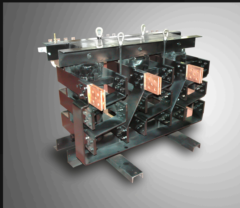
Transfo 10 000 AMPS
