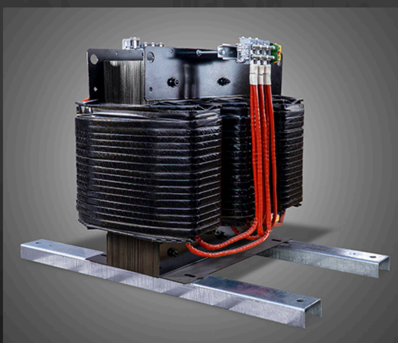
Transfo 400 Volts
