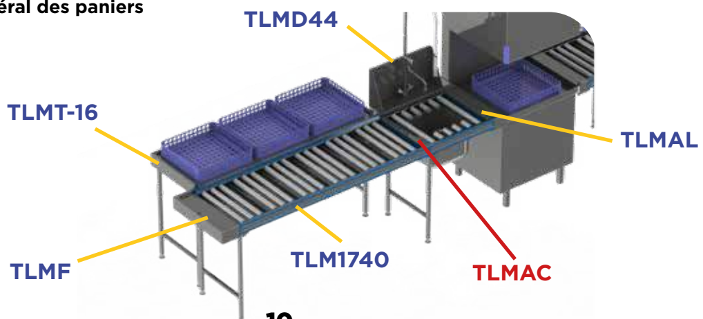
TLMT-16 raccordée à une TLM1740 pour glissement latéral des paniers
