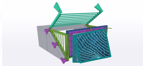
Exemple de plan de fabrication 3D de système de rétention de macrodéchets
