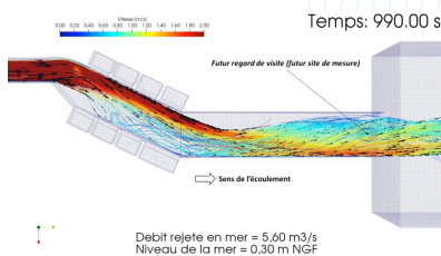
Exemple de modélisation 3D du flux
