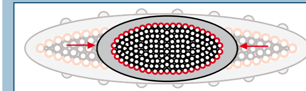
Comparaison en coupe transversale sous charge (WLL)
