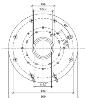
Coupe horizontale de la plaque
