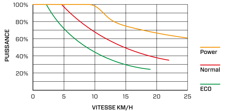
COURBE D'ACCÉLÉRATION
