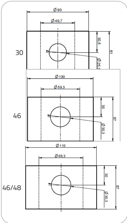
Adaptateur rotator
