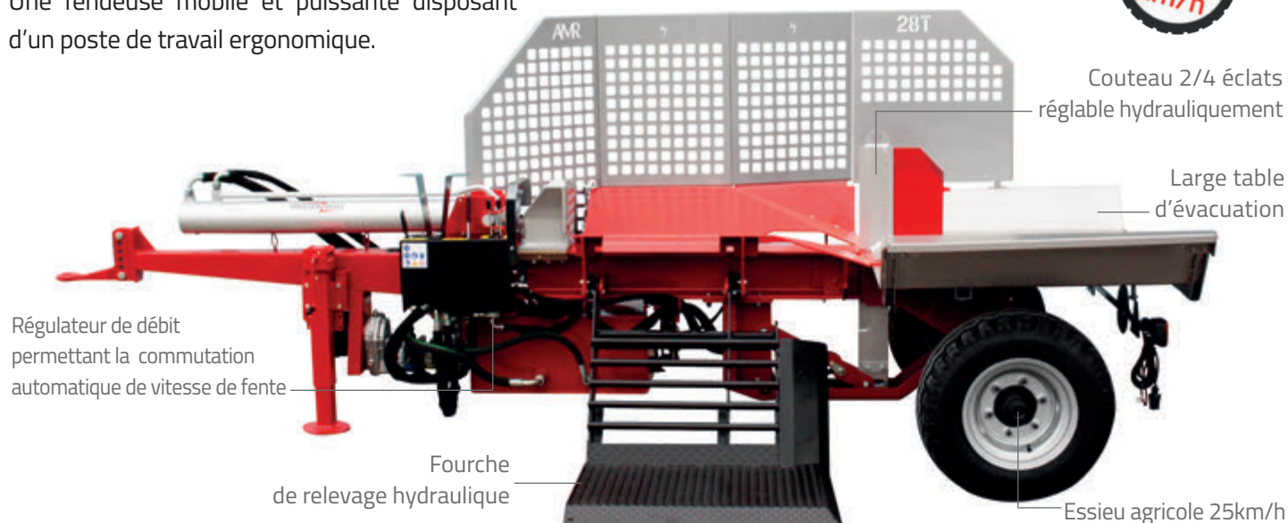
HPF28 ESS sur essieu
