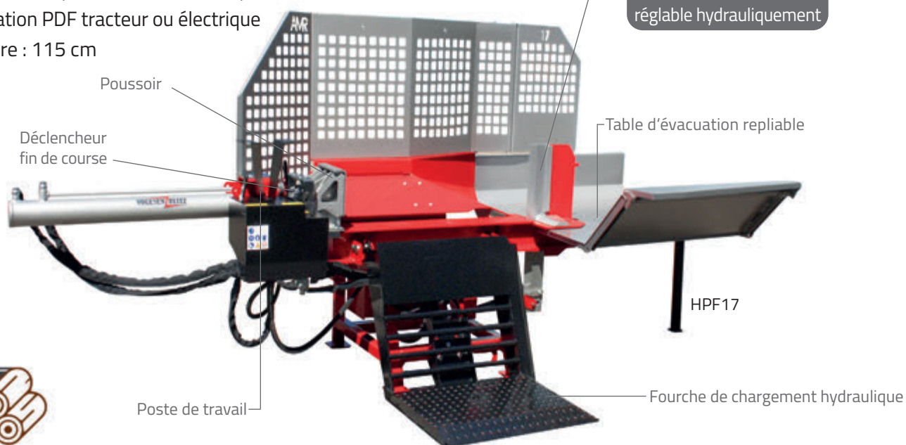
Couteau 2/4 éclats réglable hydrauliquement
