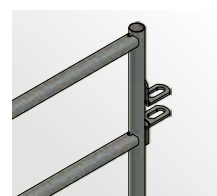
Liaison par broche avec lumières oblongues pour s'adapter au relief
