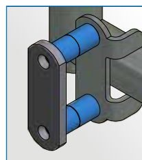
Bagues de guidage facilitant le mouvement du portillon
