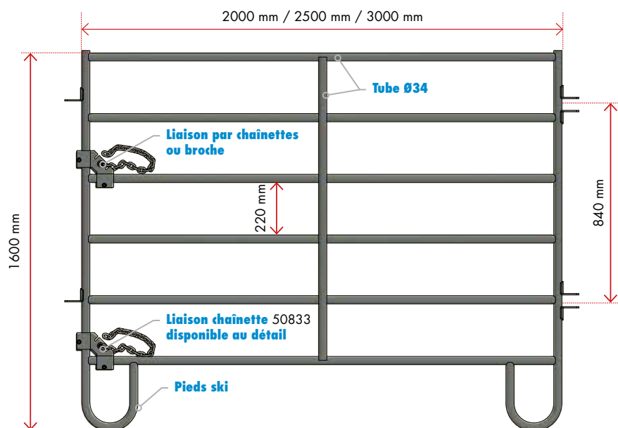
Liaison par broche avec lumières oblongues pour s'adapter au relief
