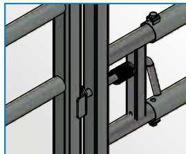
Portillon équipé d'un verrou à ressort permettant une fermeture automatique
