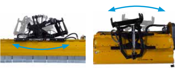
Sur un terrain irrégulier, des mouvements oscillants et de braquage généreux assurent une adaptation optimale au sol.
