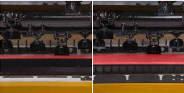
Le MU-Vario® se caractérise par une forme optimisée de l'admission et du carter, et un degré de broyage et de défibrage à réglage progressif. Pour une qualité de broyage et de défibrage idéale.
