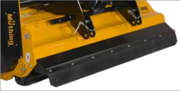
Le pare-poussière pour véhicules porteurs empêche toute entrave à la visibilité de même qu'un encrassement excessif des points d'aspiration surbaissés par la poussière dégagée.
