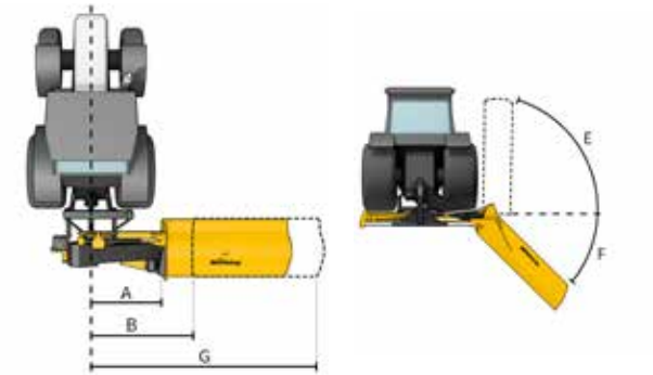
Grâce à sa conception étudiée, le broyeur MU-E/S peut être replié pour un faible encombrement d'entreposage.
