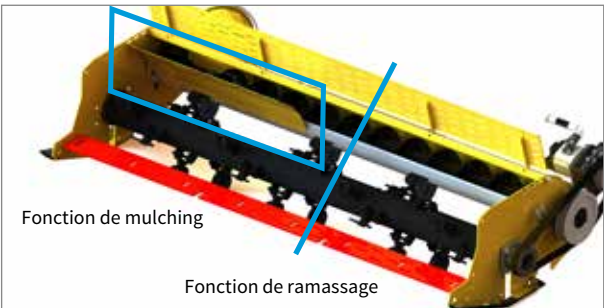
La tôle d'éjection permet de commuter entre les fonctions de ramassage et de mulching.
