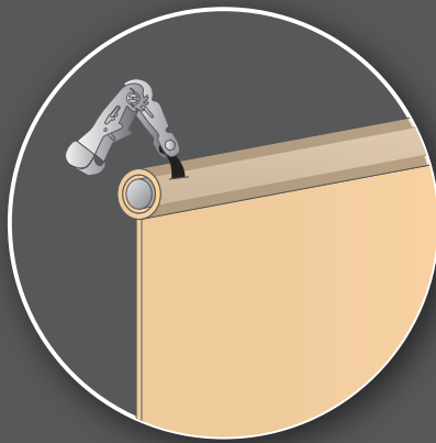
Tubes sous fourreau, avec tension par sangles à cliquets
