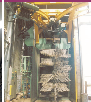
Ht 3000 - Ø 2000 mm
