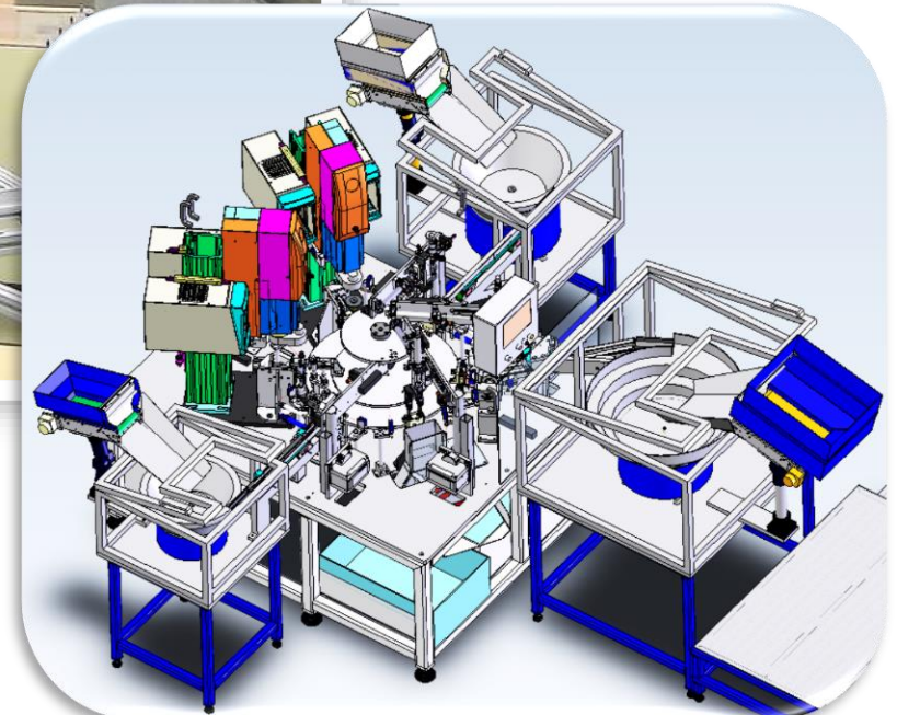
Alimentation automatique par bols vibrants
