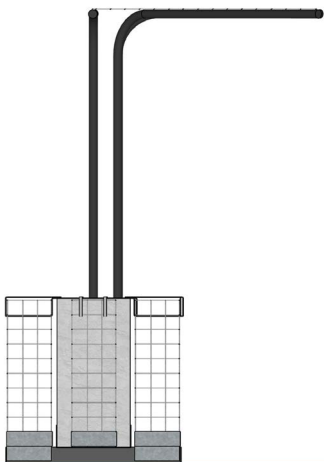
Vue de profil.
