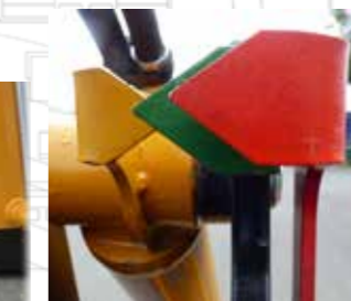
Repère de niveau et repère de position du rotor
