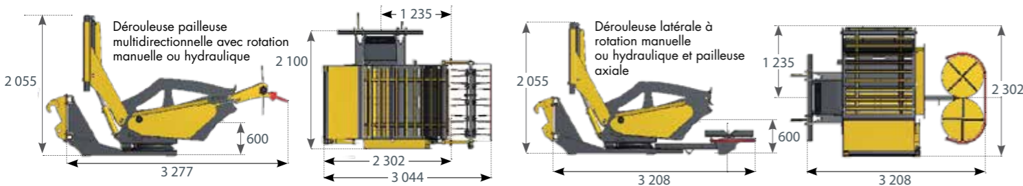
Dérouleuse pailleuse Delta avec PEIGNE
