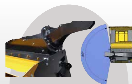
Goulotte latérale 160°. Distance jusqu'à 18 à 22 m
