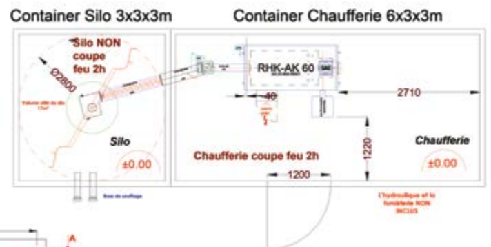
Exemple de shelter 60 kW
